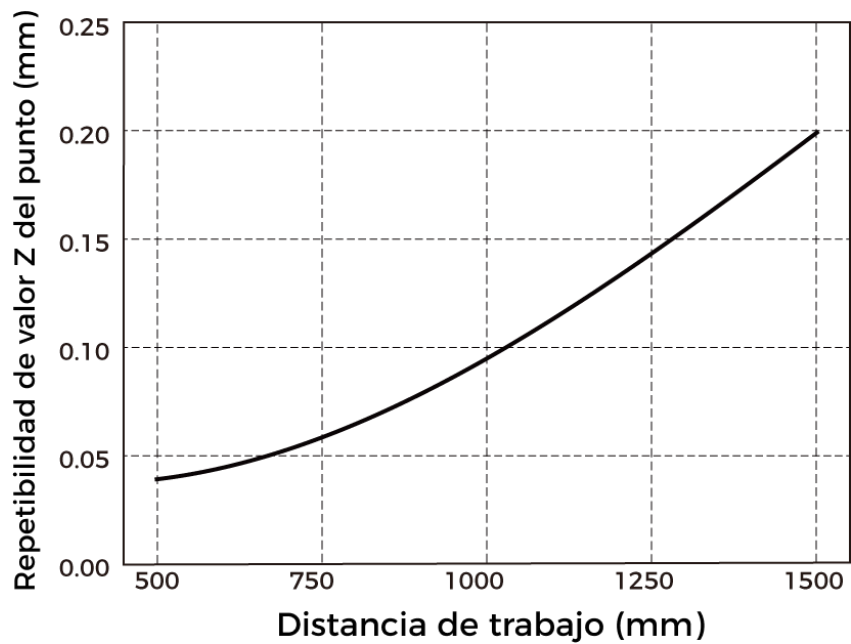
Repetibilidad de Valor Z del Punto
